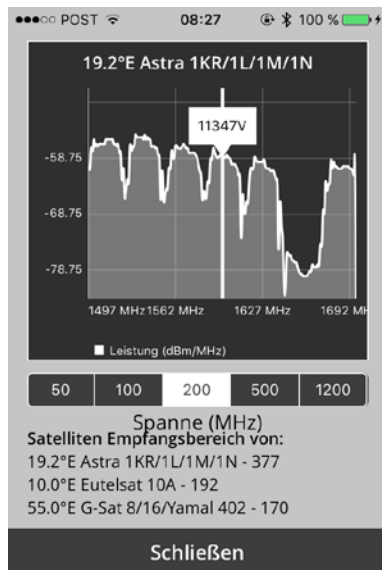
Abbildung 24: Spektrum
