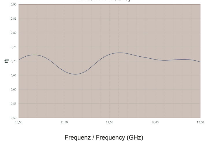
Effizienz / Efficiency
