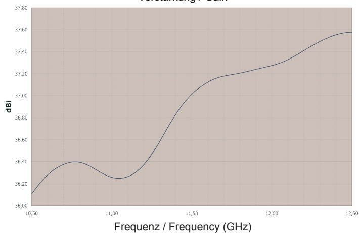
Verstärkung / Gain
